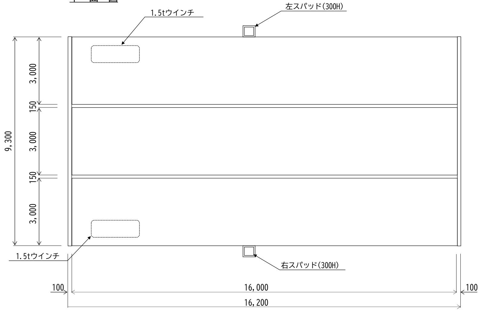
平面図
