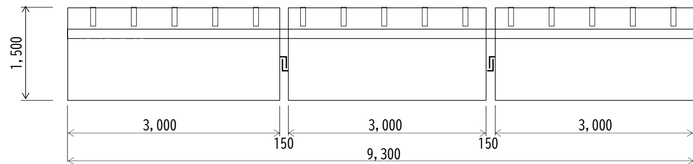
正面図
